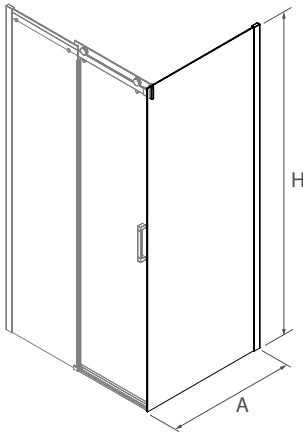
CÔTÉ FIXE SUR MESURE / par parois de douche
