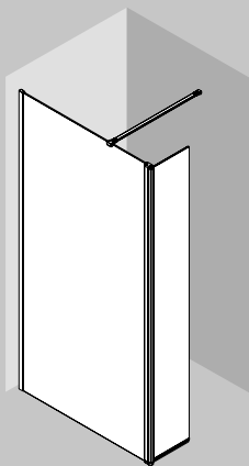
PAROI 1 FIXE + 1 VOLET PIVOTANT
